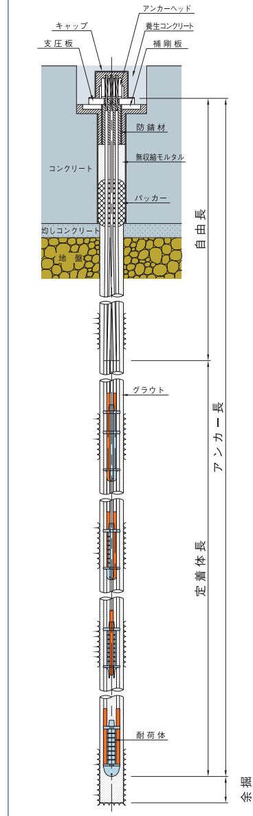
ストランドの構成 (KTB荷重分散型永久アンカーの場合)
