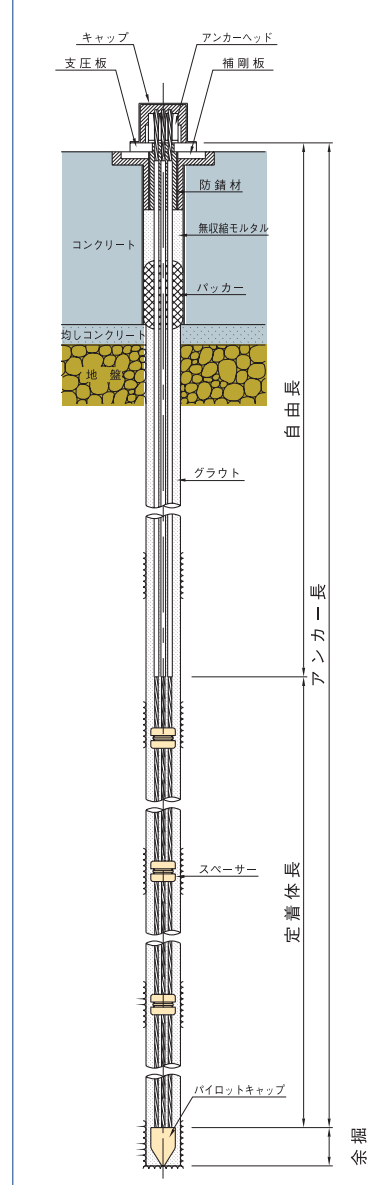
ストランドの構成 (KTB引張型SC永久アンカーの場合)
