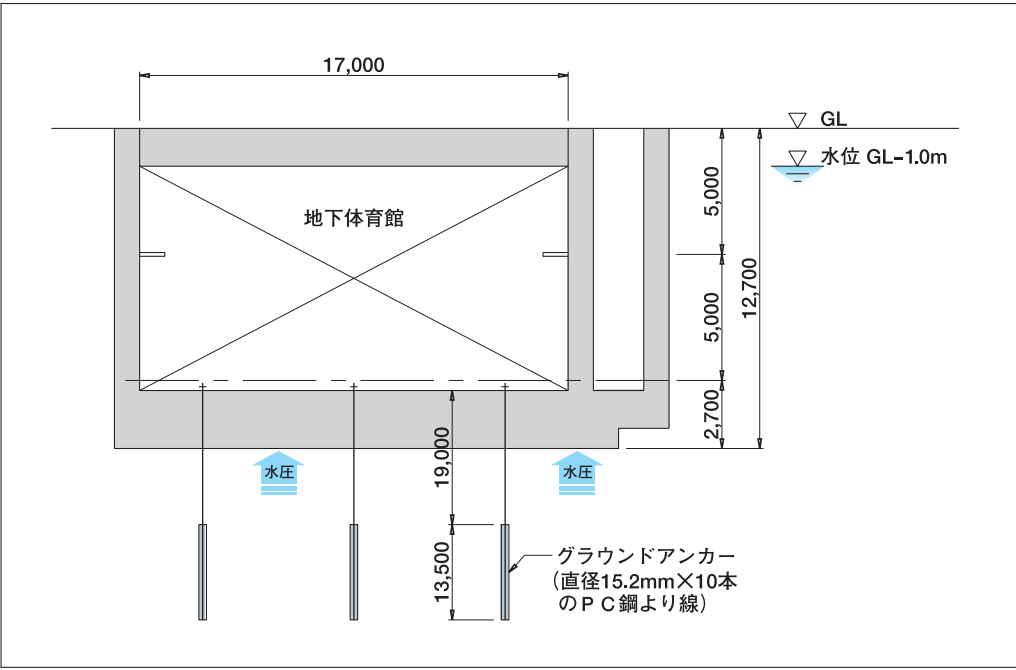
●施工イメージ図
