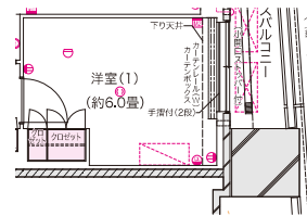
■ 11~23階部分図 SCALE:約1/150
